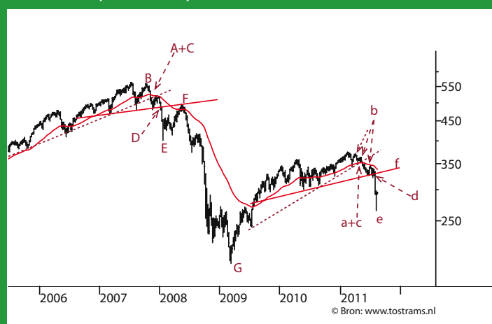
AEX INDEX (2006-2011)
